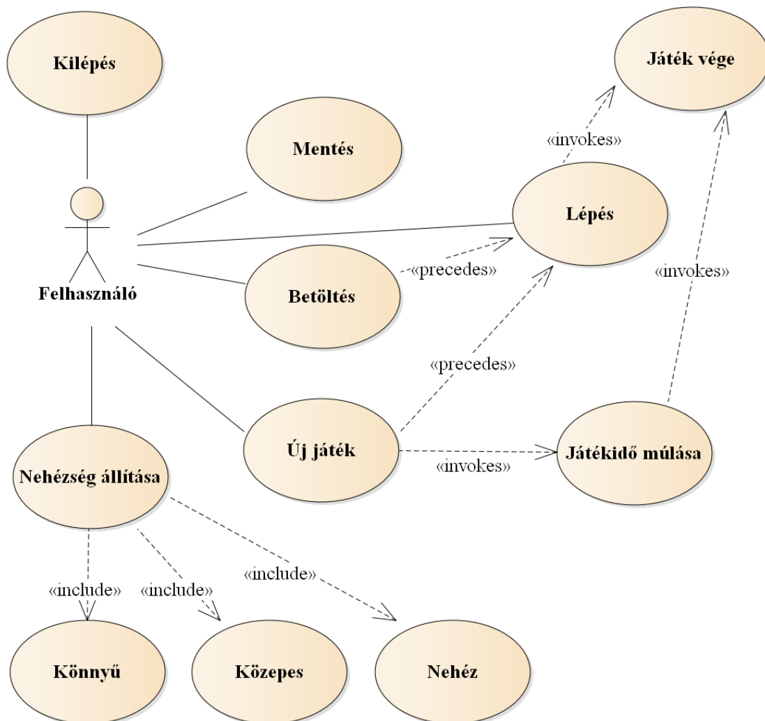
1. ábra: Használati esetek diagramja
