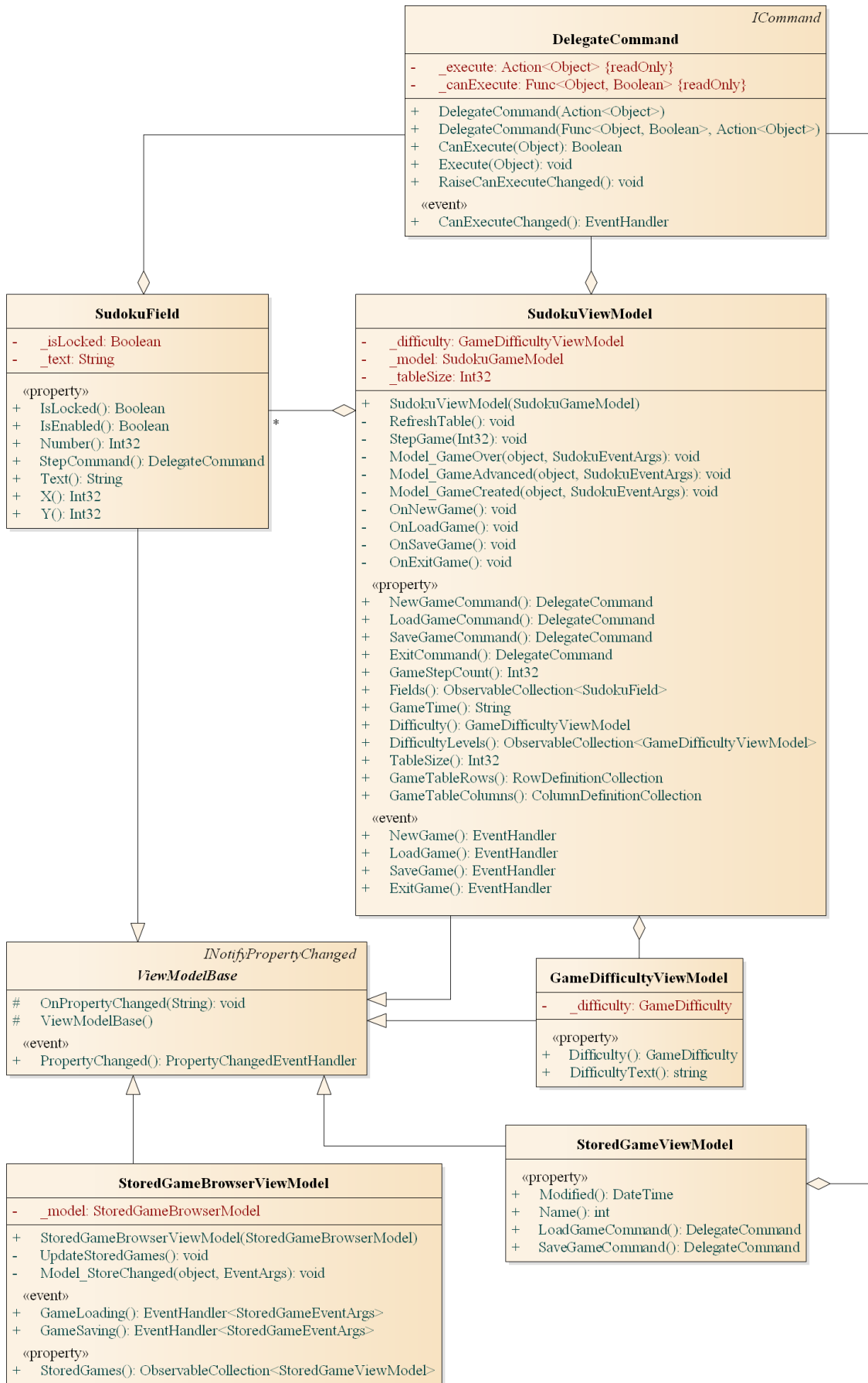
5. ábra: A nézetmodell osztálydiagramja
