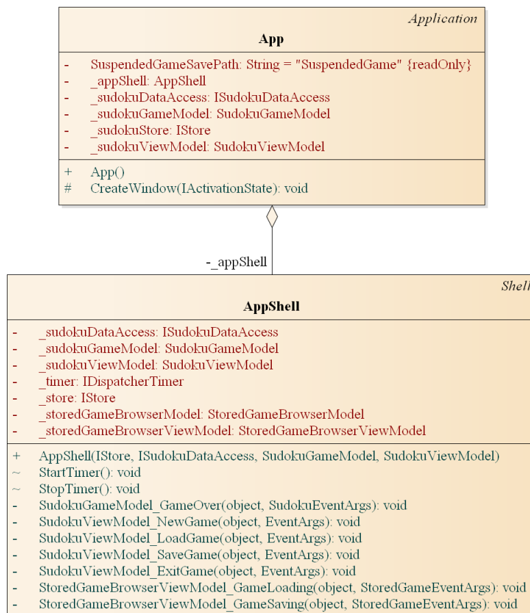
6. ábra: A vezérlés osztálydiagramja
