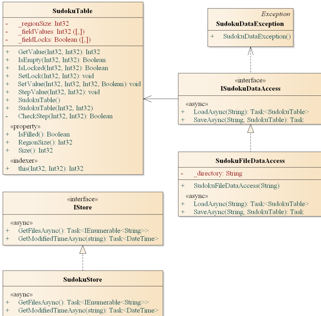
4. ábra: A Persistence csomag osztálydiagramja
