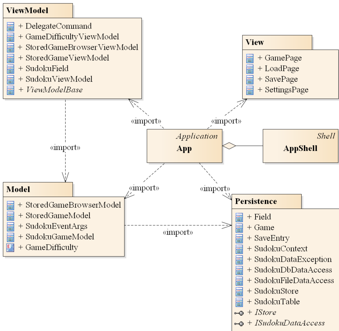
2. ábra: Az alkalmazás csomagdiagramja
