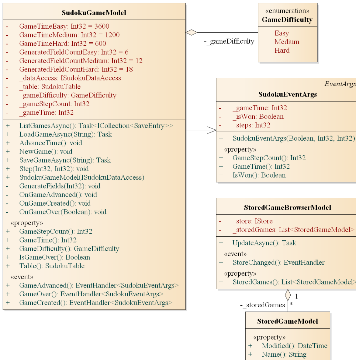
4. ábra: A Model csomag osztálydiagramja
